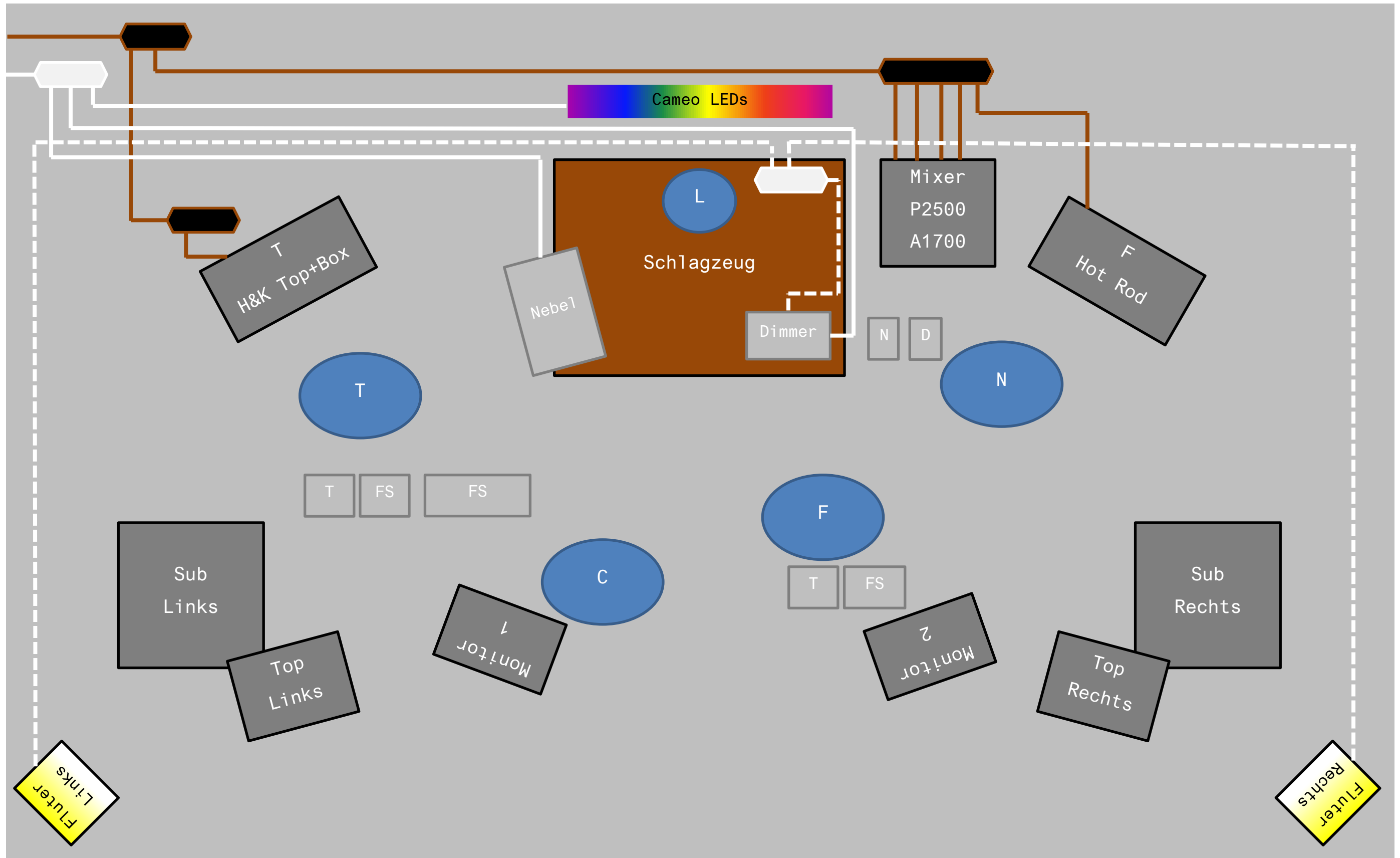
Bühnenplan mit Band-Technik bis 300 Zuhörer, Bühne ca. 5m x 4m
